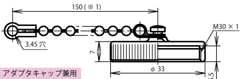
レセプタクルキャップ: NJC-28-RCa
