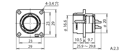
NR-20 ■ -RM
