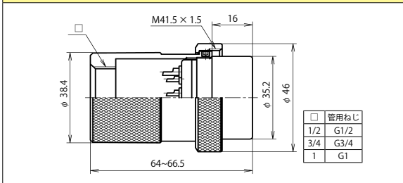
NCS-40 ■ -GP □ (注)
