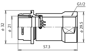
NR-24 ■ -GAdF1/2 (注)
