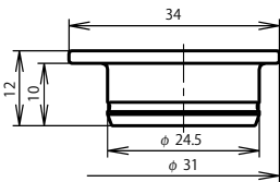
プラグキャップ：NR-24-PCa・1
