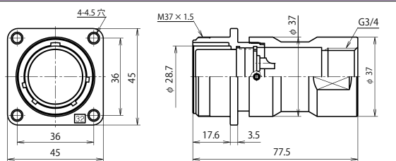
NJC-32 ■ -GAd(F)F3/4 (注)
