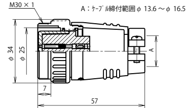
NJC-28 ■ -AdF
