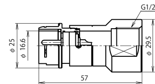
NR-20 ■ -GAdM1/2 (注)
