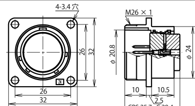
NJC-24 ■ -RM
