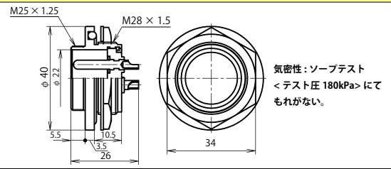
NCS-25 ■ -RBP
