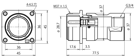
NJC-32 ■ -GAd(F)M3/4 (注)
