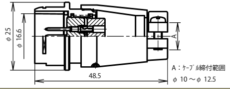
NR-20 ■ -AdM
