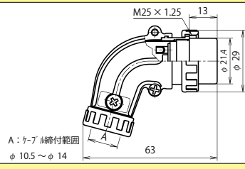
NCS-25 ■ -LP
