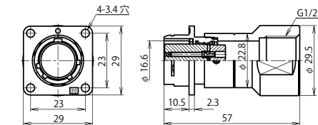
NR-20 ■ -GAd(F)F1/2 (注)
