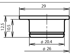
プラグキャップ: NR-20-PCa・1
