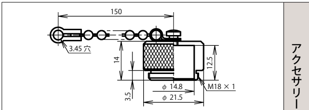
プラグキャップ: NCS-16-PCa
