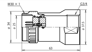
NJC-28 ■ -GAdM3/4 (注)
