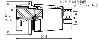
NR-24 ■ -AdF
