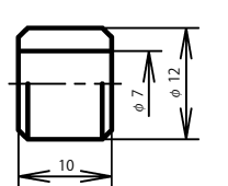
ケーブルブッシング: CBAS-12-7
