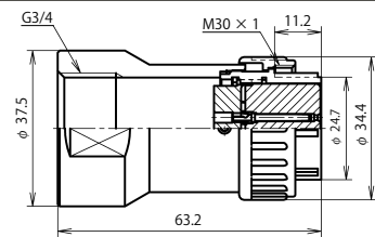
NJC-28 ■ -GPF3/4 (注)
