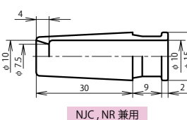
ケーブルブッシング: NJC-20-CB
