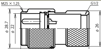
NCS-25 ■ -GAd1/2 (注)
