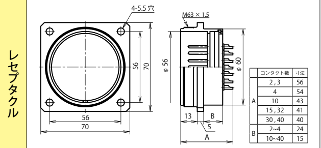
NCS-60 ■ -R
