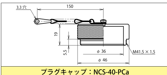
プラグキャップ：NCS-40-PCa
