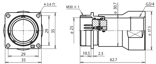
NJC-28 ■ -GAd(F)M3/4 (注)
