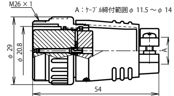
NJC-24 ■ -AdF
