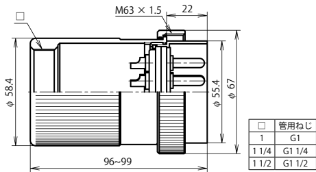
NCS-60 ■ -GPM □ (注)
