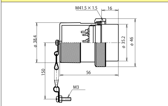
NCS-40 ■ -SP
