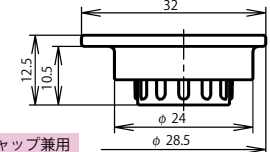
レセプタクルキャップ：NR-20-RCa・1
