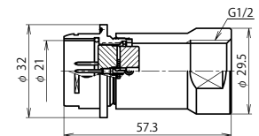
NR-24 ■ -GAdM1/2 (注)
