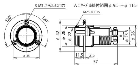
NCS-25 ■ -Ad(F)
