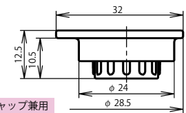
レセプタクルキャップ：NR-20-RCa・1
