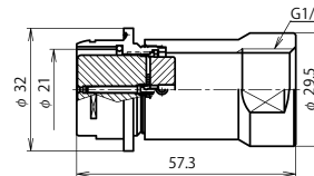
NR-24 ■ -GAdF1/2 (注)
