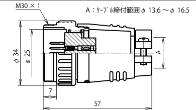
NJC-28 ■ -AdM
