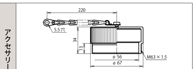
プラグキャップ：NCS-60-PCa
