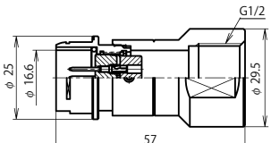
NR-20 ■ -GAdM1/2 (注)
