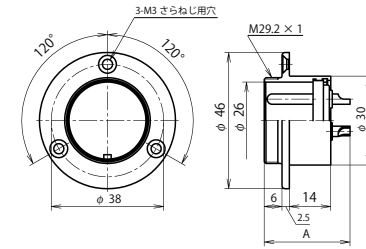
NCS-30 ■ -R
