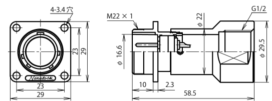
NJC-20 ■ -GAd(F)M1/2 (注)
