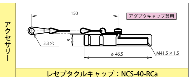
レセプタクルキャップ：NCS-40-RCa
