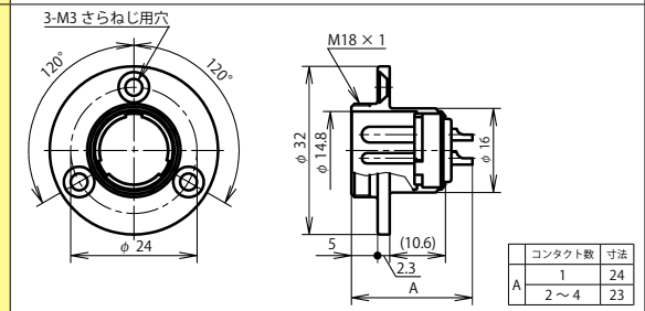
NCS-16 ■ -R-CH
