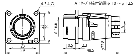
NR-20 ■ -Ad(F)F
