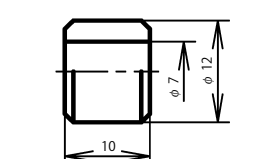
プラグ, アダプタ用
