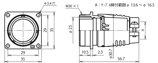
NJC-28 ■ -Ad(F)F
