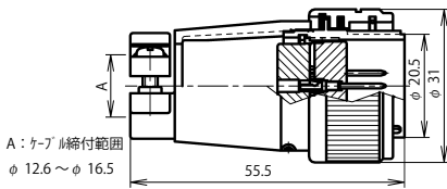
NR-24 ■ -PM
