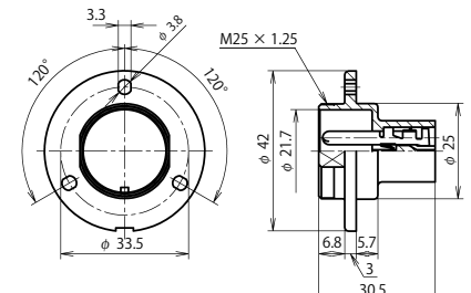
25AA-■RM
