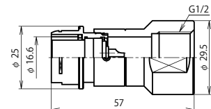
NR-20 ■ -GAdF1/2 (注)
