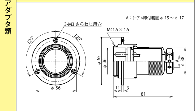
NCS-40 ■ -Ad(F)
