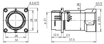
NR-24 ■ -GAd(F)M1/2 (注)
