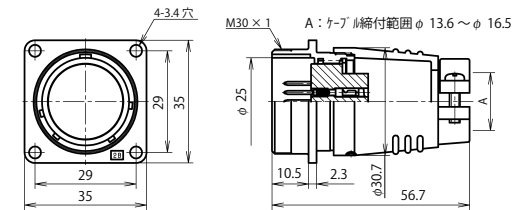
NJC-28 ■ -Ad(F)M
