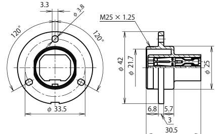
25AA-■RF
