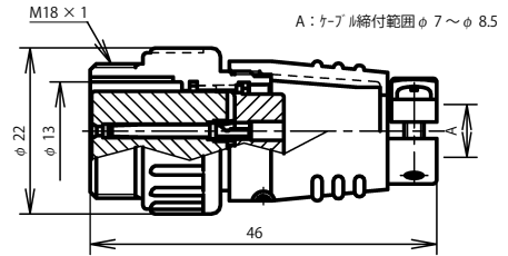
NJC-16 ■ -AdF
