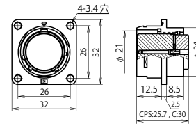
NR-24 ■ -RF
